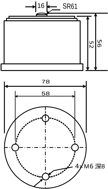
安装方式 Working Diagram
